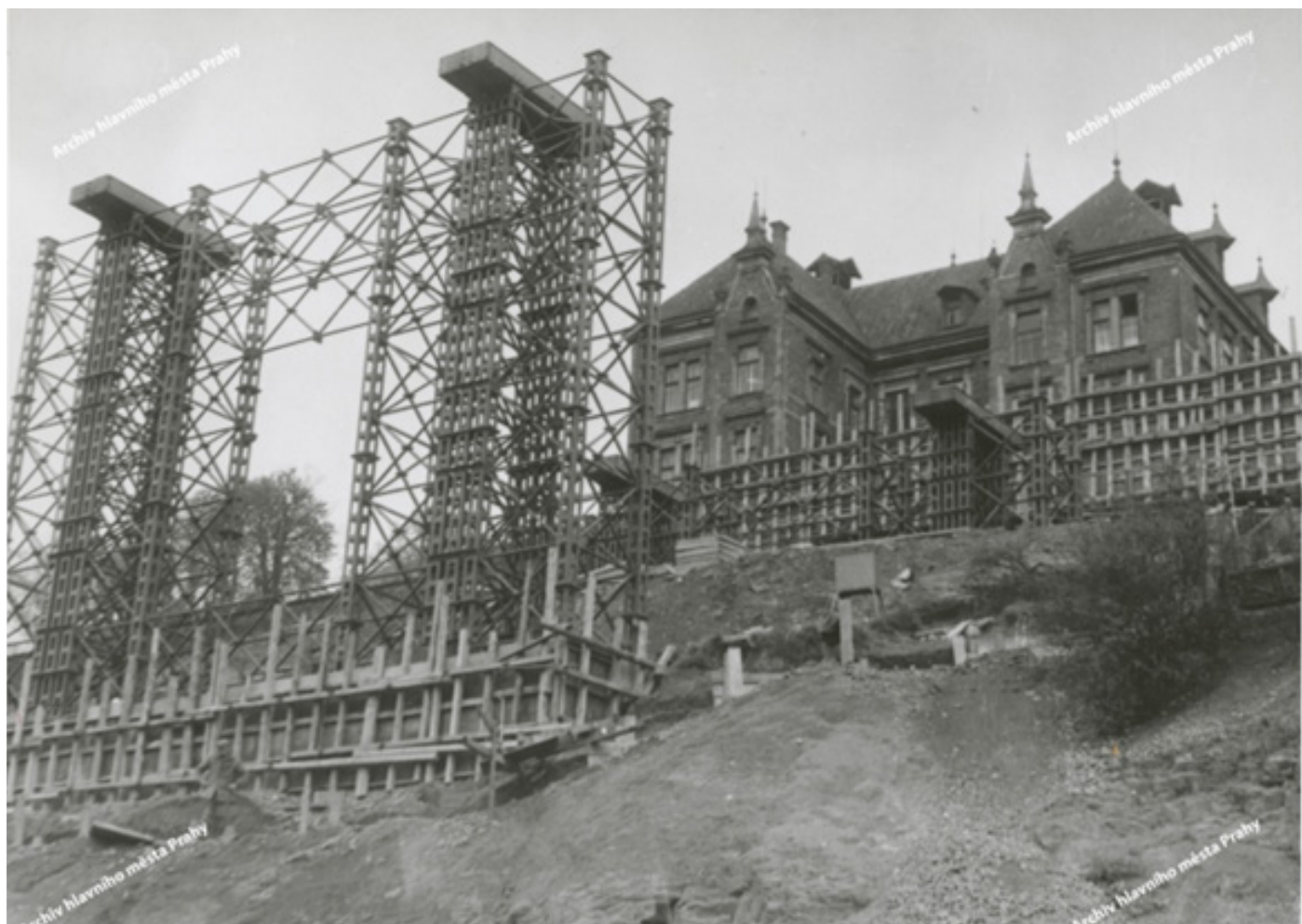
Stavba Nuselského mostu. Pomocné skruže na novoměstské straně. V pozadí dům čp. 1962 (Česká dětská nemocnice). Foto Václav Mikšátko, 1966.
